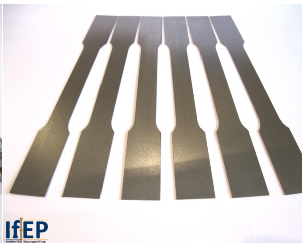
Flachproben
